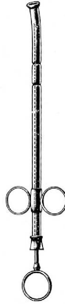
RAPID BI 29-8115-01 200 x 8mm BI 29-8115-02 250 x 10mm BI 29-8115-03 250 x 12mm
