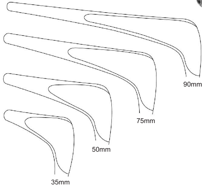
BI 22-6617-35 BI 22-6617-50 BI 22-6617-75 BI 22-6617-90
