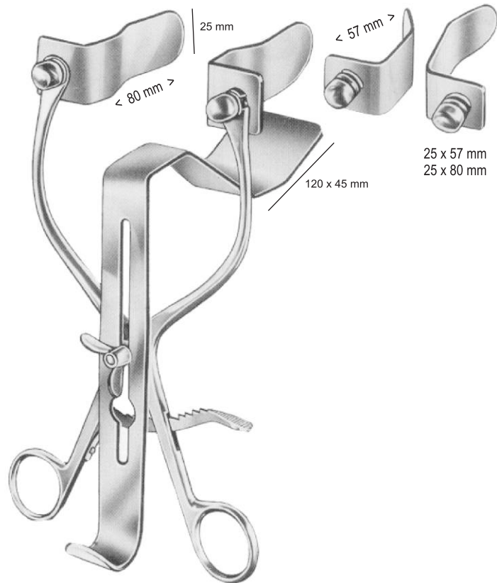
MILLIN BI 16-4804-25
