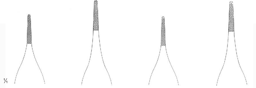
BI 09-2301-12 12 cm/4 3/4" 0.4 mm BI 09-2301-15 15 cm/5 7/8" 0.4 mm BI 09-2302-12 12 cm/4 3/4" 1 x 2 0.4 mm BI 09-2302-15 15 cm/5 7/8" 1 x 2 0.4 mm
